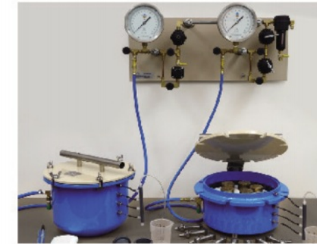
토양보수력(pF)측정기
